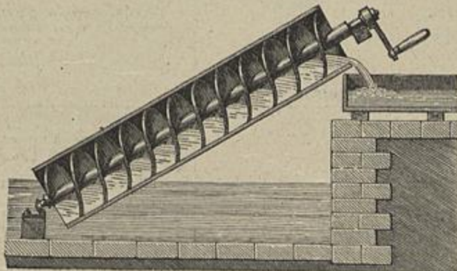
Fig. 31 — Parafuso de Archimedes
