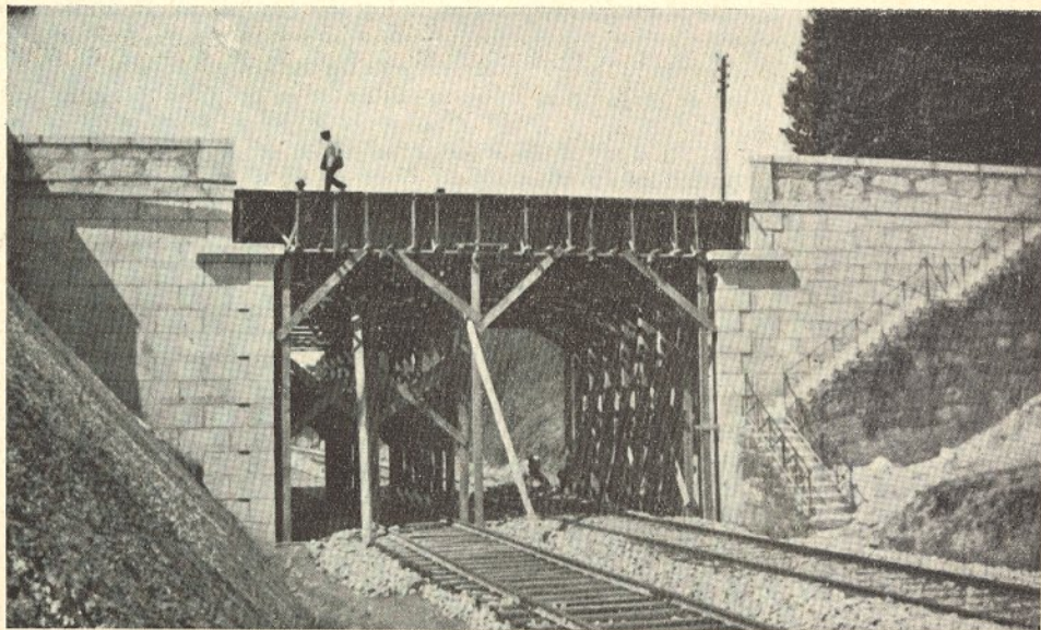
LINHA DE CIRCUNVALAÇÃO DO PORTO — Passagem da Palmilheira (em construção)
