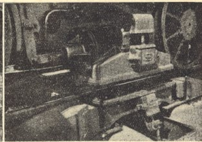
Figura 3—Eléctro-íman da locomotiva passando sobre um eléctro-íman da via.
