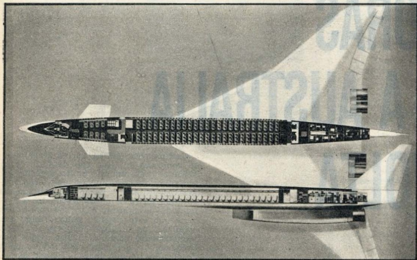
DOIS CORTES LONGITUDINAIS (SEGUNDO DIFERENTES PERSPECTIVAS) DO PROJECTO NORTE-AMERICANO SST, QUE CONSTITUI UMA VERSÃO MELHORADA DO CÉLEBRE BOMBARDEIRO XB 70, DESTINANDO-SE EMBORA À AVIAÇÃO CIVIL
