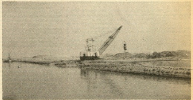
Uma draga gigante procede ao alargamento do Canal
