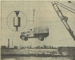
CAMION DE 2 1/4 TONELADAS SUSPENSO POR 2 CILINDROS DE AÇO COM 10 CMS. DE DIÂMETRO 'COLADOS' COM P LIOBOND
