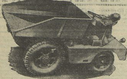
DUMPER «JUNG» Tipo K 40 Capacidade 3m3 = 6 ton.
