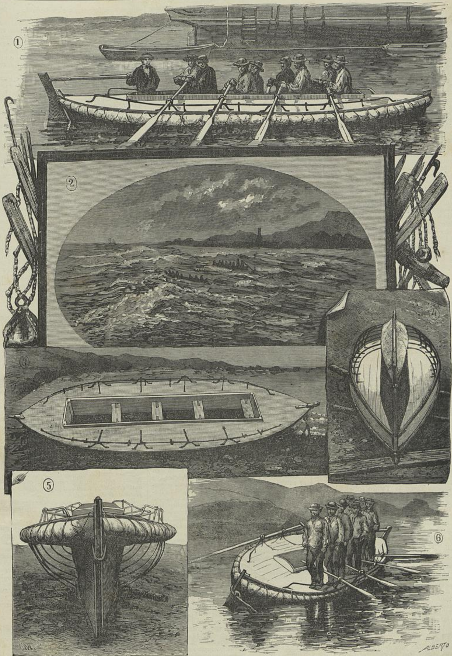
SALVA-VIDAS RELVAS (Segundo photographias de Carlos Relvas) 1 VISTA DE PERFIL. — 2 SALVA-VIDAS RELVAS NA EXPERIENCIA OFFICIAL. — 3 VISTA DE PLANTA. — 4. VISTA DE QUILHA. — 5 VISTA DE PROA. 6 PRIMEIRA EXPERIENCIA.
