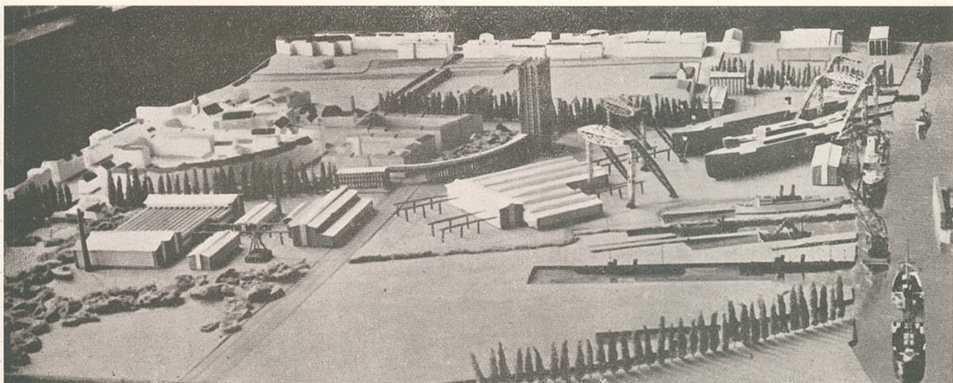
Projecto do novo estaleiro «Vulcano», de Stettin, cuja primeira pedra foi lançada há dias. Este estaleiro havia sido desmantelado por imposição do Tratado de Versalhes. Ali se construiram antes da guerra barcos de grande tonelagem. Agora vai ressurgir, servindo, ao mesmo tempo, de local de instrução para a arquitectura naval alemã.
