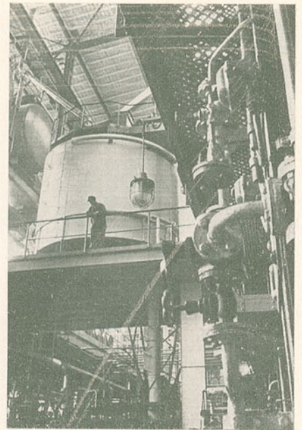
Trecho de uma fábrica de produção de borracha sintética
