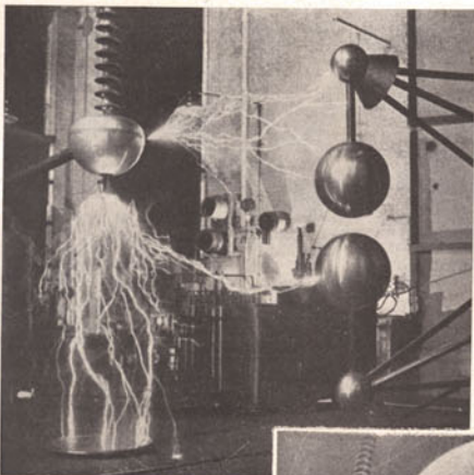
Em cima: Curioso aspecto duma descarga de 200.000 volts. À direita: O condensador empregado na medição das altas voltagens
