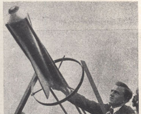
O inventor alemão Gerhard Zucker realizou há dias experiências de transporte de correio por meio de foguetões entre Hampshire e a ilha de Wight. A experiência não deu resultado mas o inventor não se dá por vencido.
