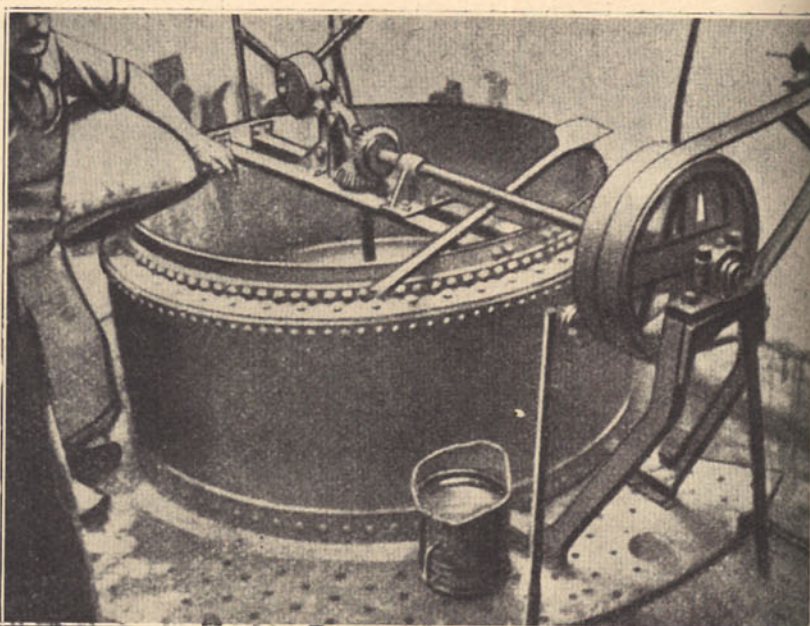
Caldeira onde se efectua a inversão do açúcar de cana, munida de um grande agitador
