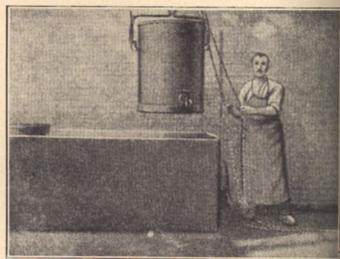
Processo de esfriar o açúcar invertido pela imersão das marmittas em água fria
