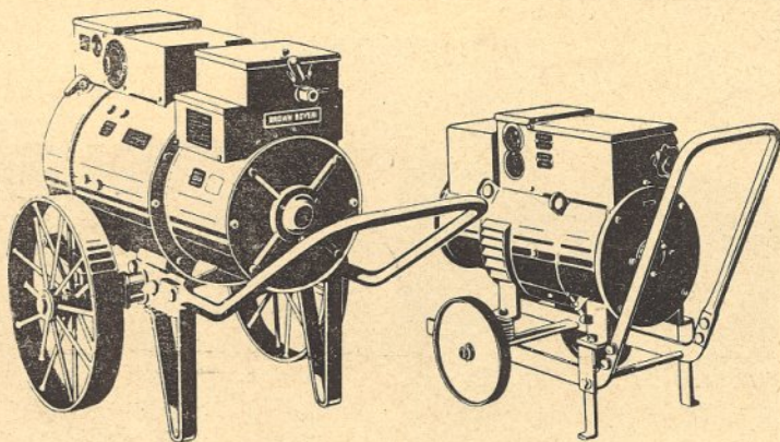
Grupos transportáveis para a soldadura eléctrica pelo arco :: :: em corrente continua de 80-180 A e 240-500 A :: ::
