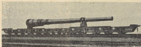
Vagão especial com 24 rodas, destinado ao transporte de cargas de grande tonelagem. A gravura mostra-nos um desses vagões, carregado com uma peça naval com 18 m ,90, pesando 105 toneladas
