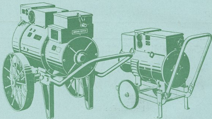
Grupos transportáveis para a soldadura eléctrica pelo arco :: :: em corrente continua de 80-160 A e 240-500 A :: ::
