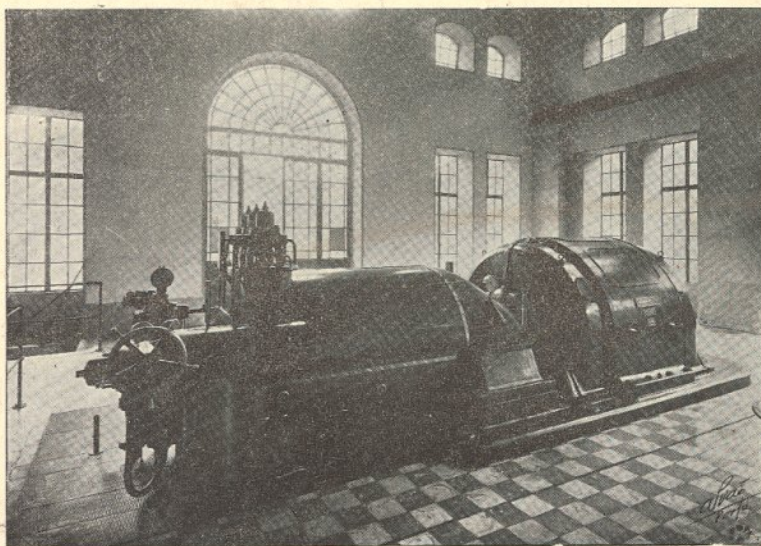
Turbo-grupo a vapor BROWN-BOVERI de 6400 kilowatts na central termica de Caniços da Companhia Hidro-Electrica do Varosa
