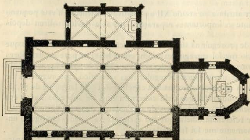
Capella de St.º André — Planta
