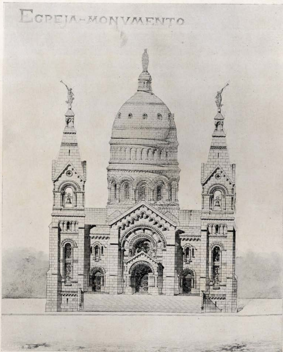
Projecto d'uma egreja monumento
