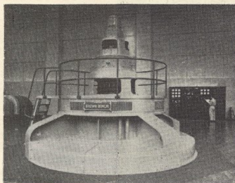
Alternador de 6000 KVA na Central de Paradelá
