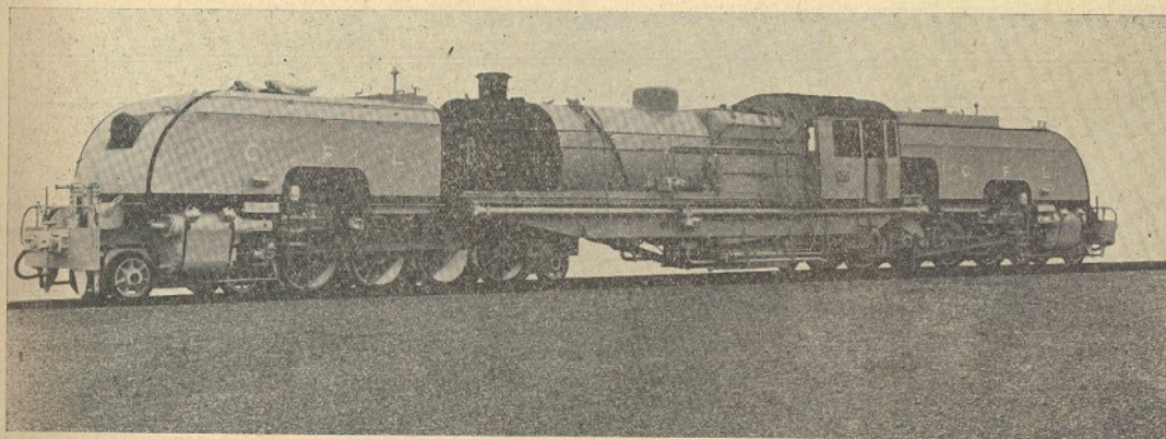
VISTA LATERAL DA LOCOMOTIVA BEYER-GARRATT
