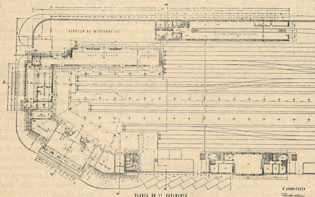
Planta do Primeiro Pavimento
