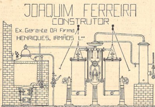
APARELHO DISTILADOR DE BAGAÇO
