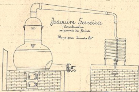
Alambiques para bagaços, vinhos e figos, a fogo directo
