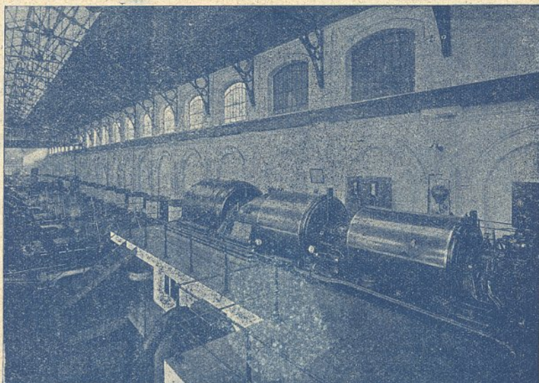
||| p o r t o O turbo grupo a vapor de 5.000 kilowatts da Central de Massarelos da Companhia Carris de Ferro do Porto
