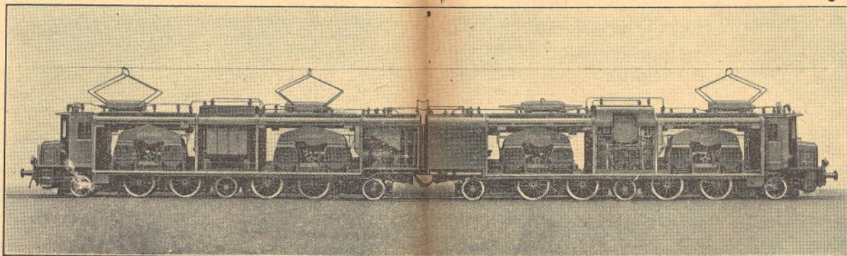
A locomotiva eléctrica de 8.800 H.P., dos Caminhos de Ferro Federais Suíços, com os painéis laterais levantados
