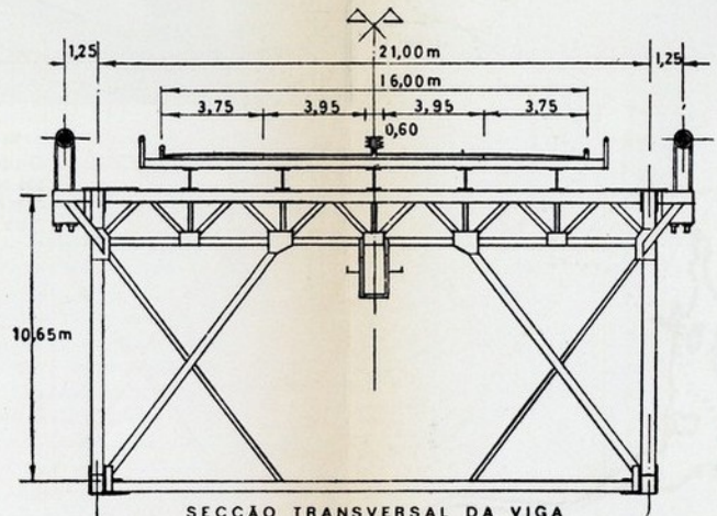
SECCÃO TRANSVERSAL DA VIGA
