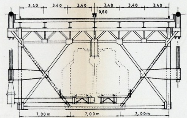
SECCÃO TRANSVERSAL DA VIGA
